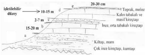
Şekil 3. Büyük Karaağaç tepenin güney yönünden alınmış kesit (ölçeksiz).
