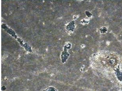
Şekil 9. Kireç çamurtaşı. Erime boşluklu (siyah lekeli alanlar) olup boşluklar kısmen kalsitle doldurulmuştur. Kaya gözenekli yapı gösterir (Büyütme: 10x).
