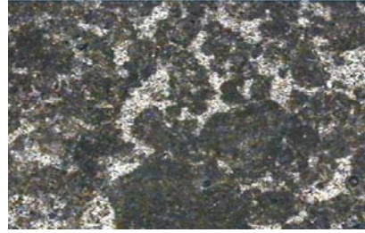
Şekil 7. Peloidli, kireç çamurtaşı dokusunda kireçtaşı. Örnek boşluklu olup, boşluklar tamamen kalsitle doldurulmuştur. Kayada gözeneklilik bulunmamaktadır (Büyütme: 10x).
